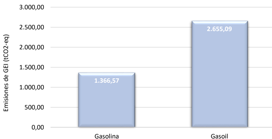
Gráfica 8. Emisiones asociadas al transporte privado y comercial en Tejeda (tCO 2 -eq). Año 2012
