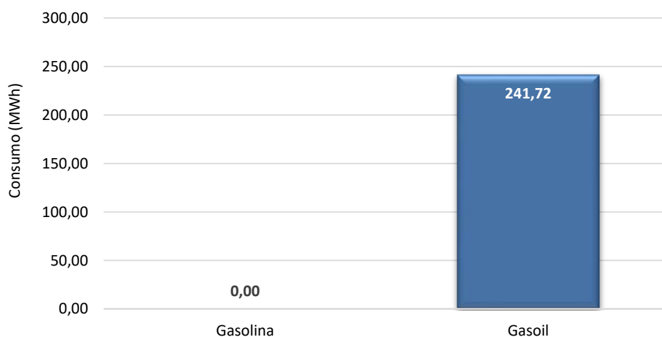
Gráfica 5. Consumo de combustibles de la flota municipal de vehículos en Valleseco (MWh). Año 2012
