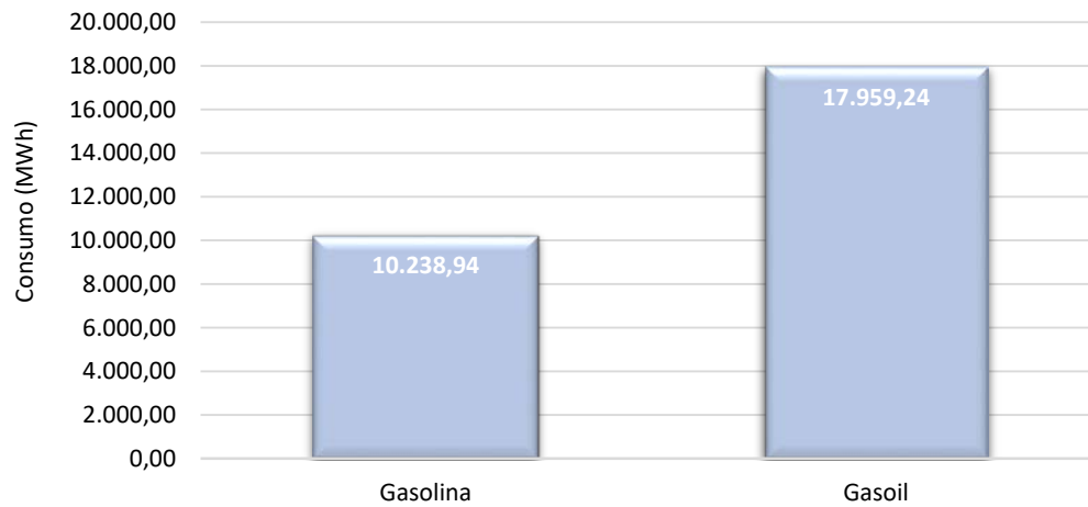
Gráfica 7. Consumo de combustibles del transporte privado y comercial en Valleseco (MWh). Año 2012
