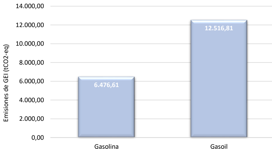
Gráfica 8. Emisiones asociadas al transporte privado y comercial en Valsequillo de Gran Canaria (tCO 2 -eq). Año 2012
